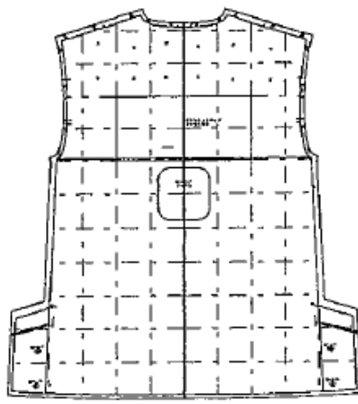
後身頃 表地x1
